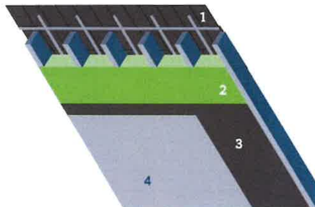
1. Onderdak | 2. Isolatie | 3. Dampschermbaan | 4. binnenafwerking
