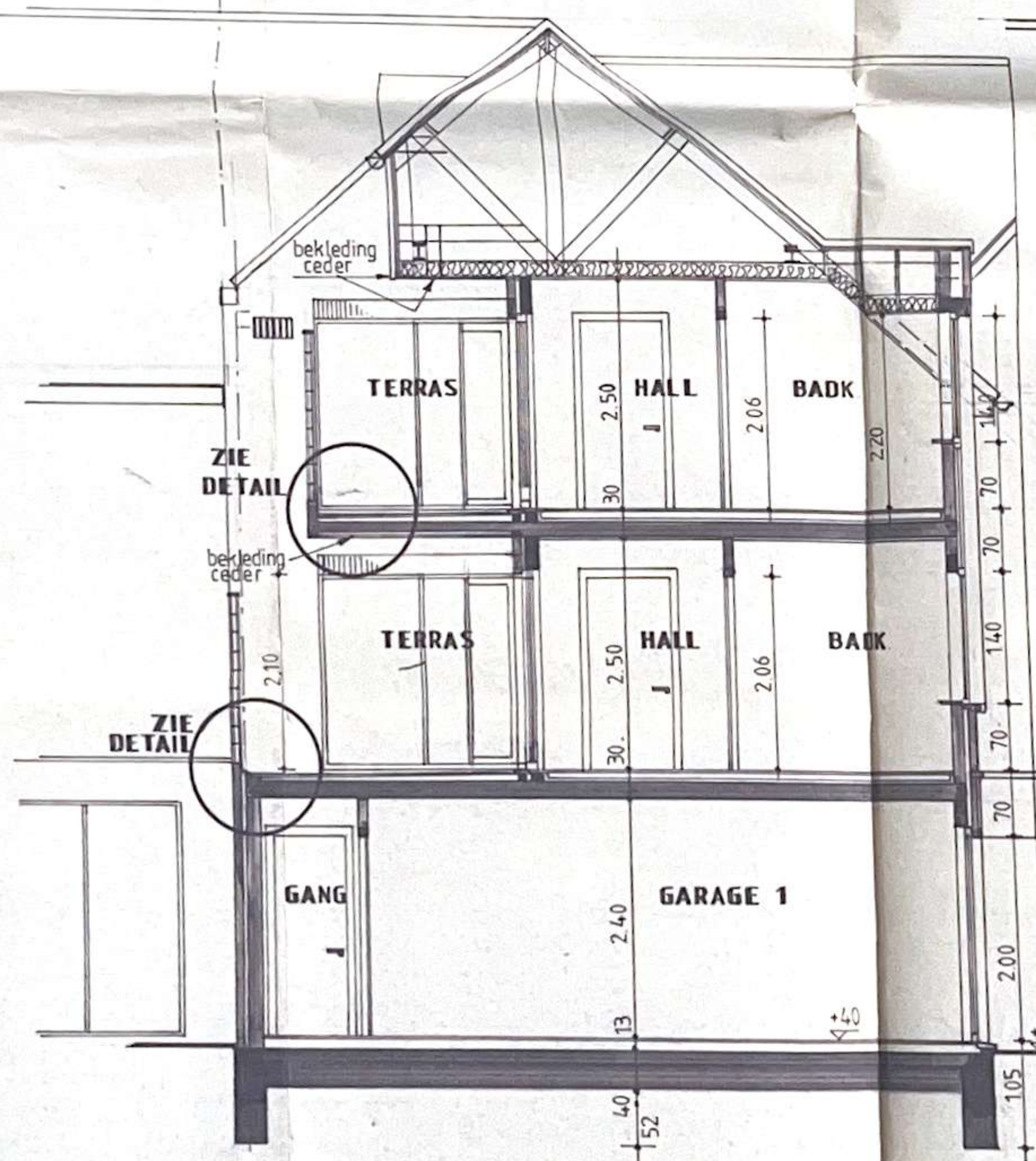
doorsnede ab
