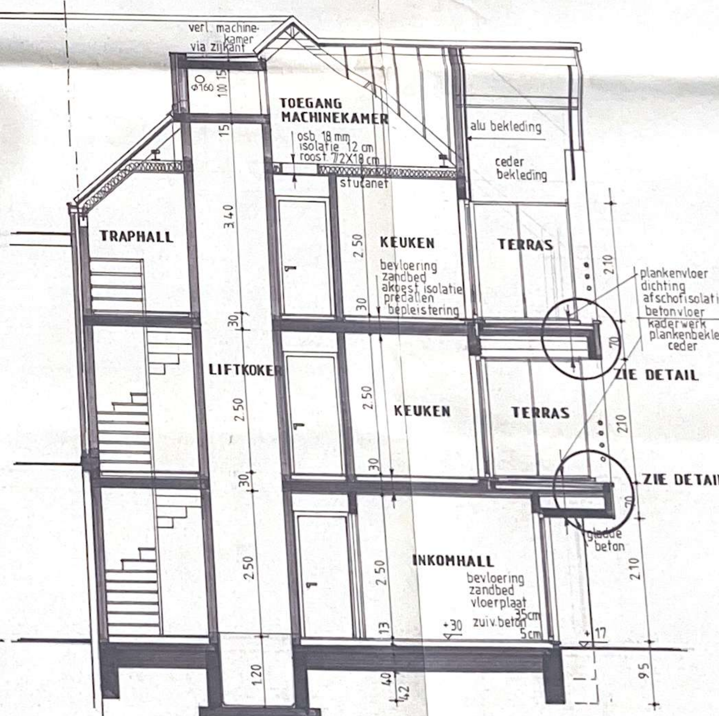
doorsnede cd.
