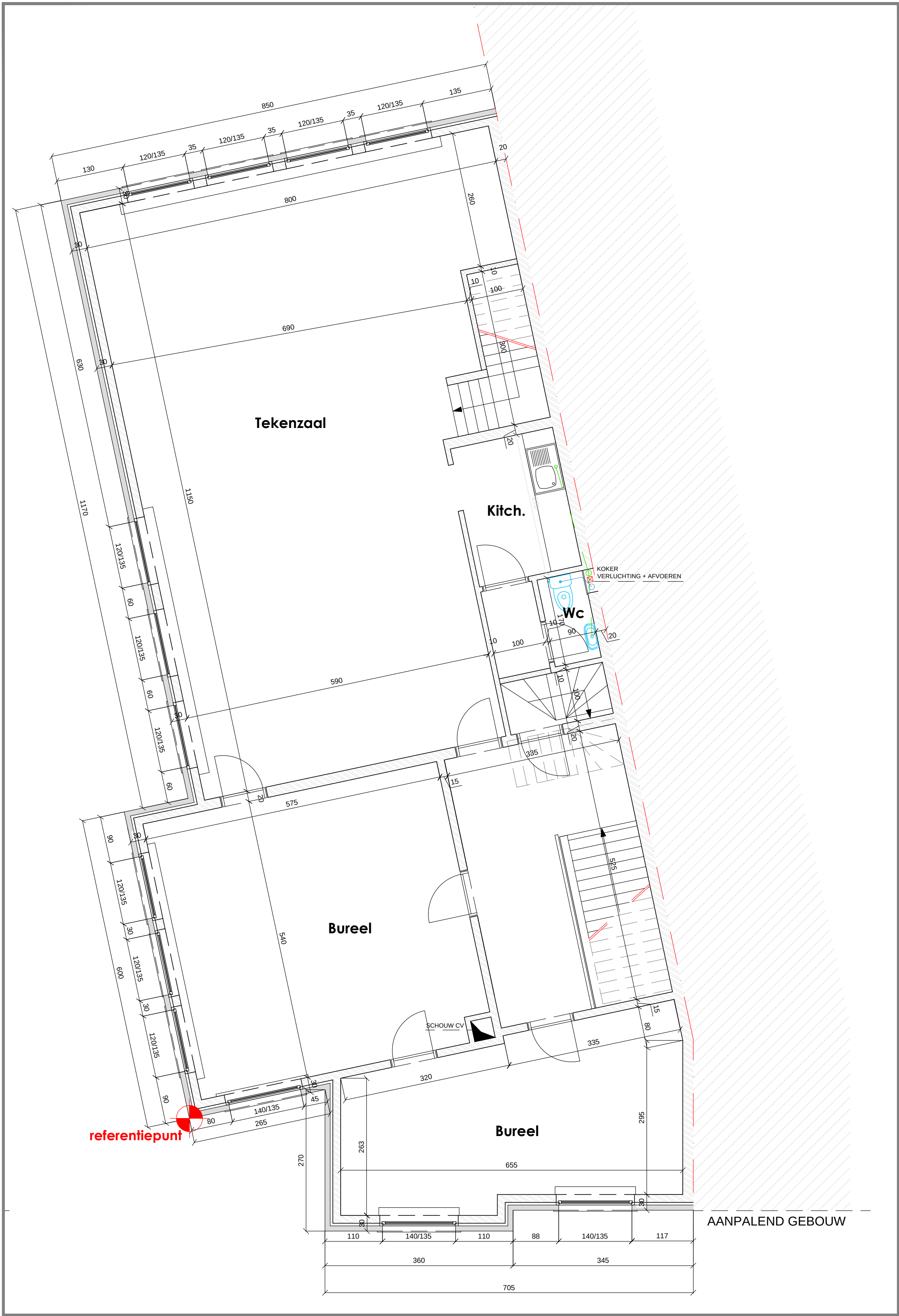
NIVEAU +1 BUREEL BESTAAND
