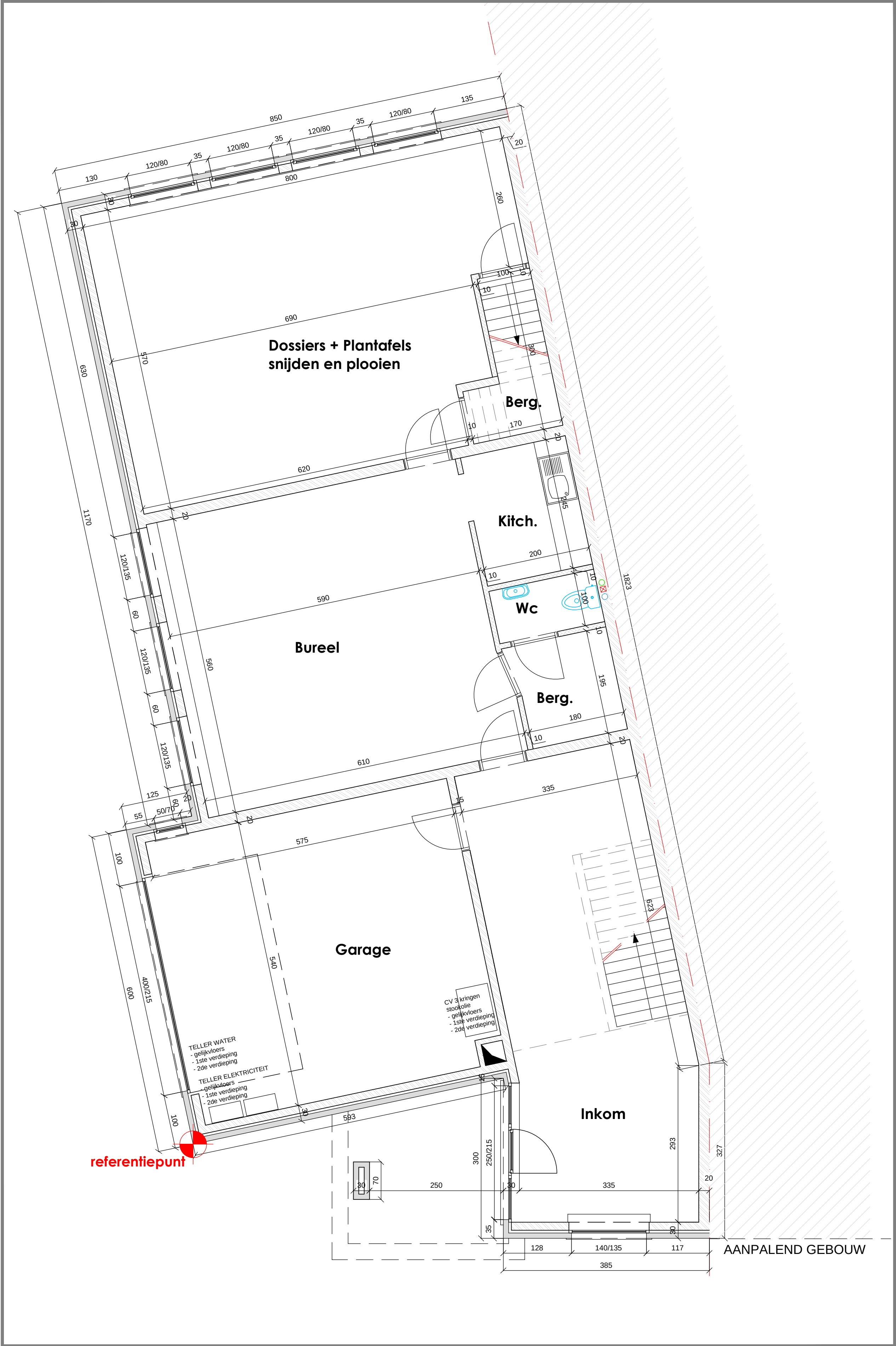
GRONDPLAN BUREEL BESTAAND
