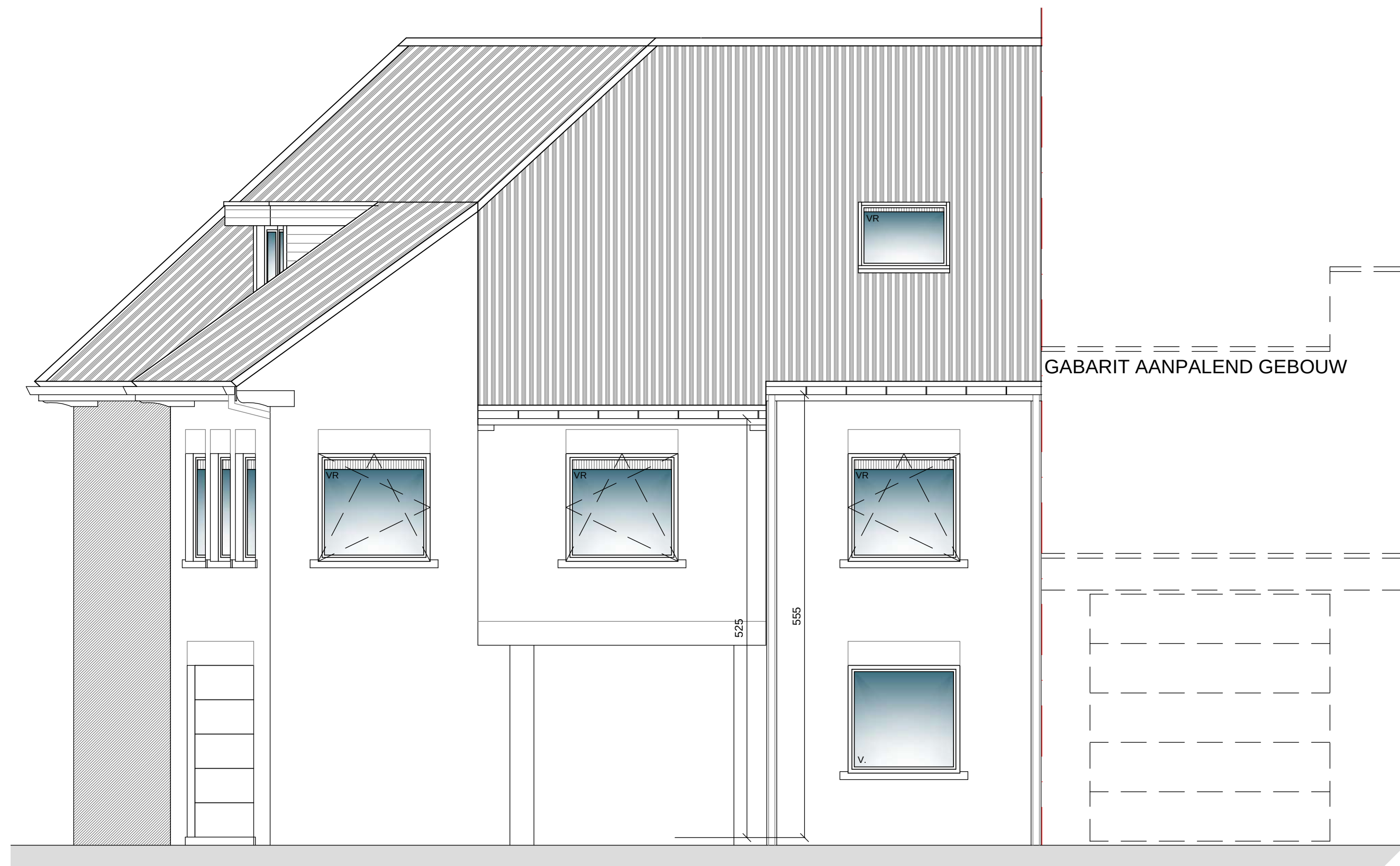
VOORGEVEL nieuw
