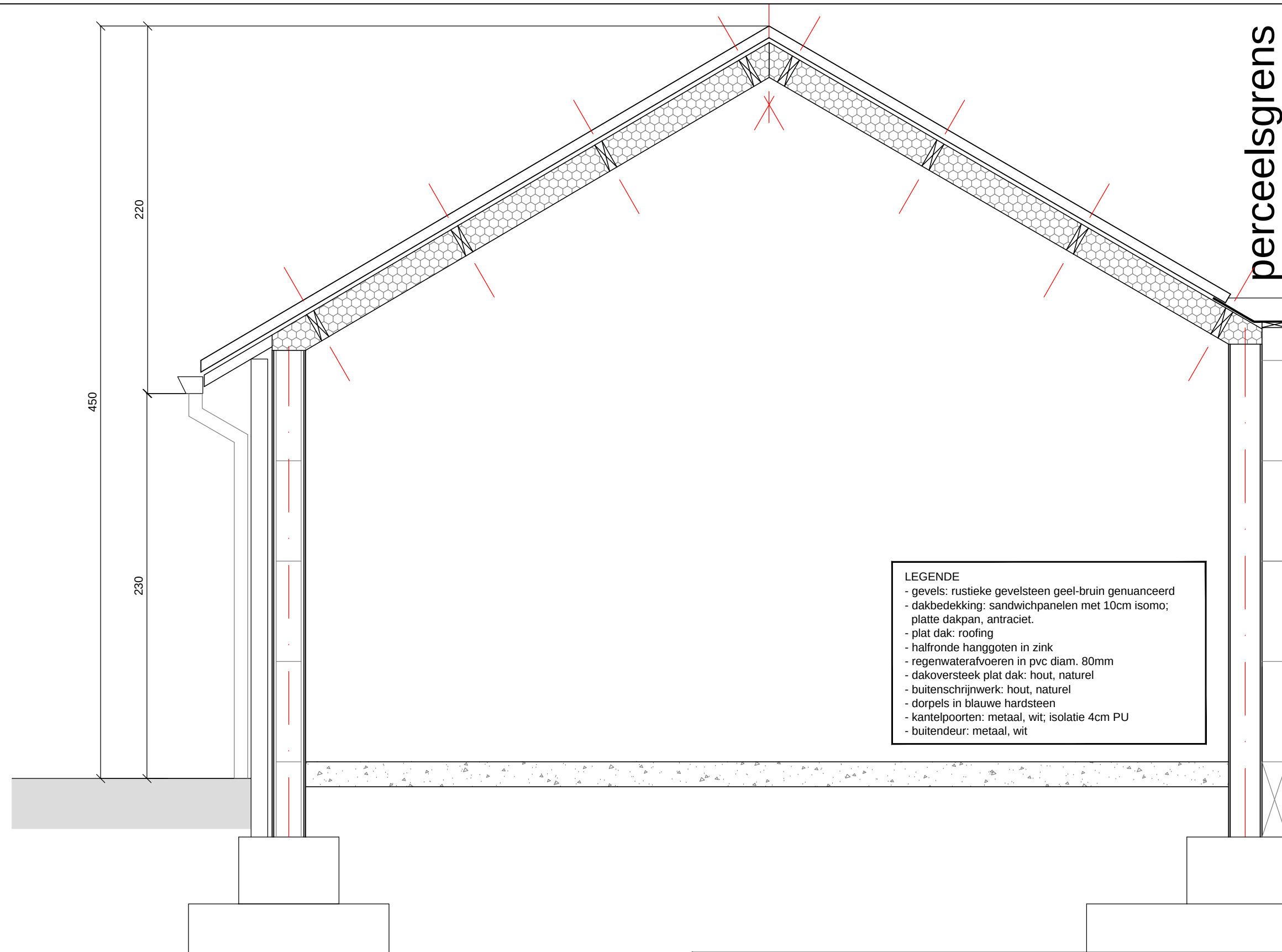
DOORSNEDE GARAGE/BERGING
