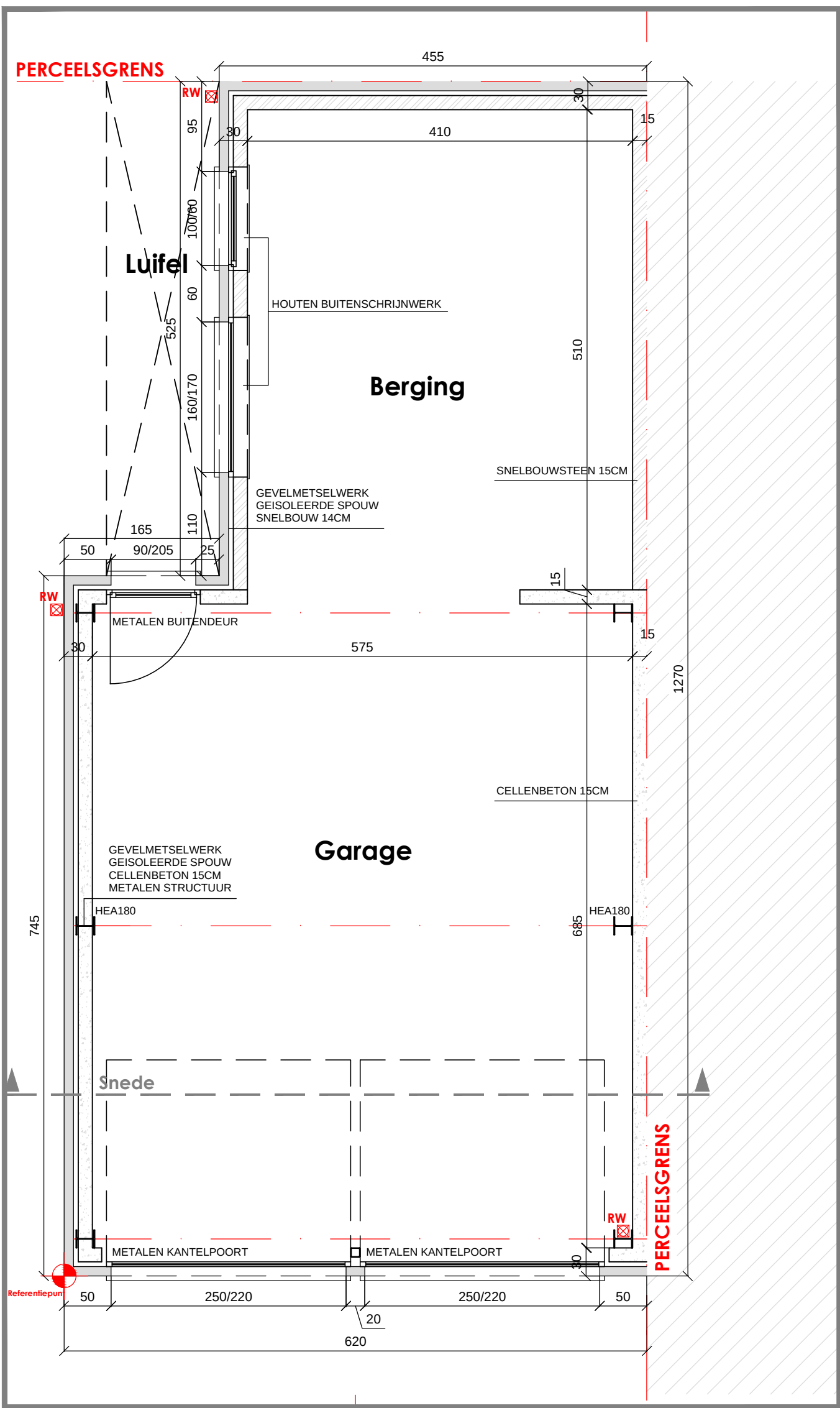
GRONDPLAN GARAGE / BERGING
