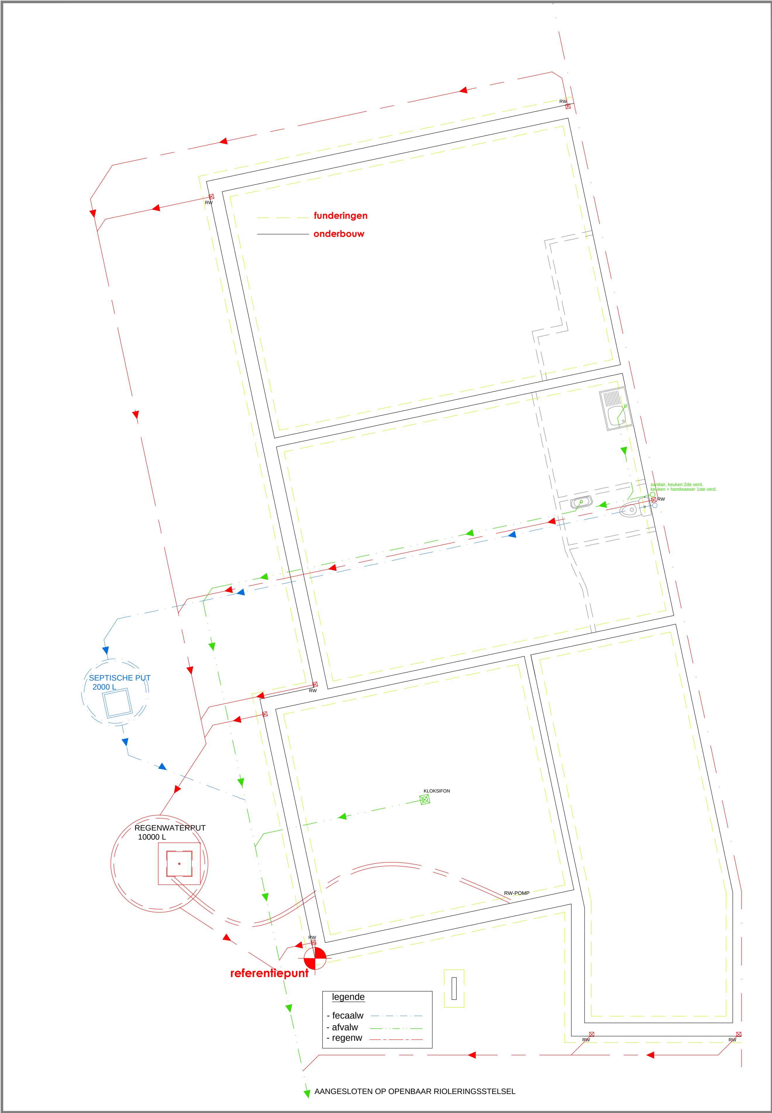
FUNDERING RIOLERING BESTAAND
