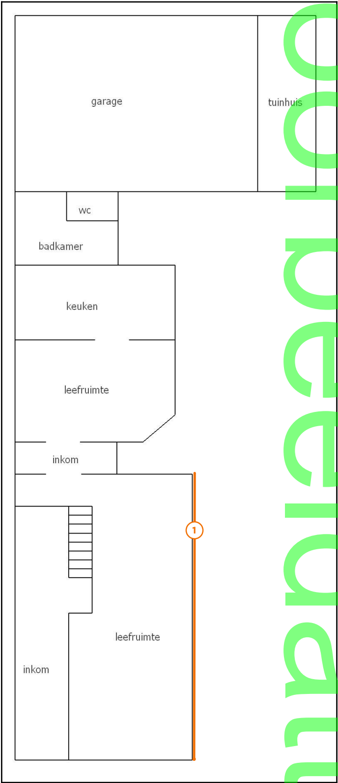
Legende van plan 1.8: grondplan gelijkvloers
