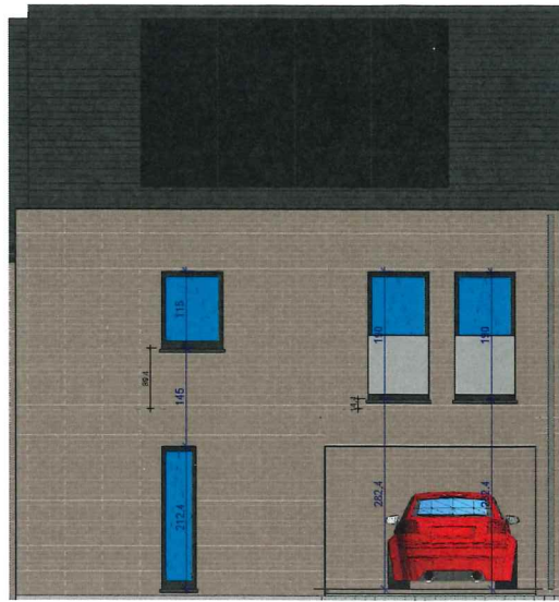
6 Voorgevel lot 186 VK 1: 50
