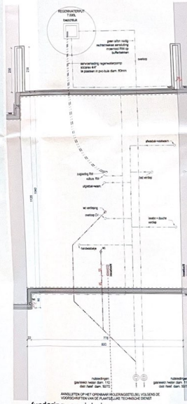
2 fundering- en rolering 1:50
