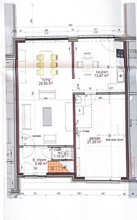
3 gelijkvloers 1:50
