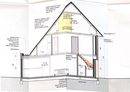
8 doorsnede 1:50
